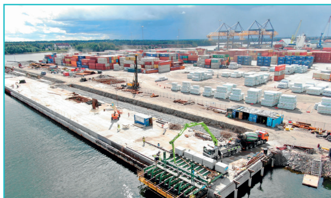
Gävle Hamn med pågående utbyggnad.
